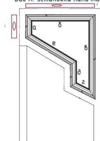
Модуль Г Вид А. Установка наличника
