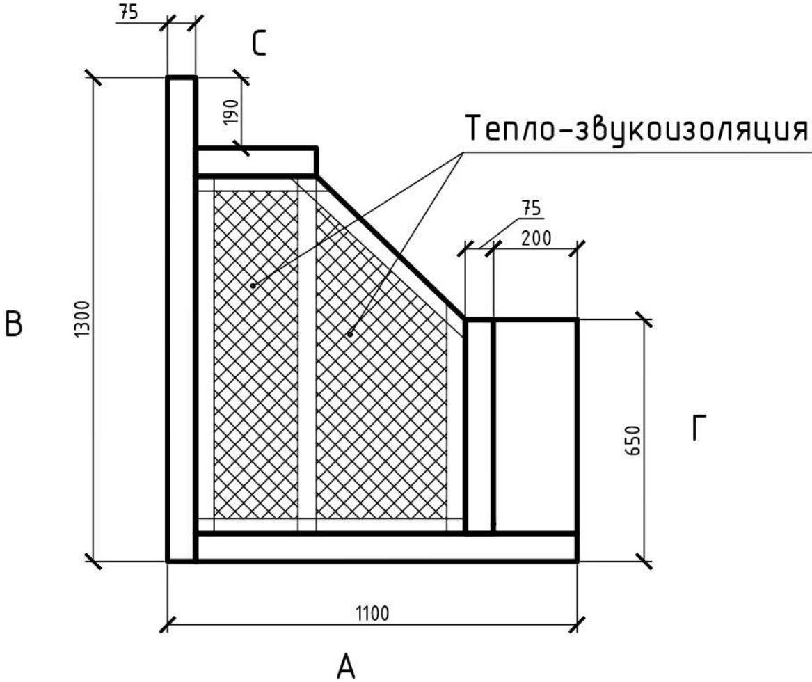
Вид сверху
